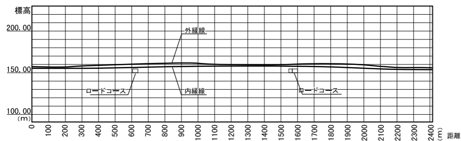
オーバルコース縦断図
